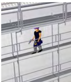
1 Ponteggio per facciate
